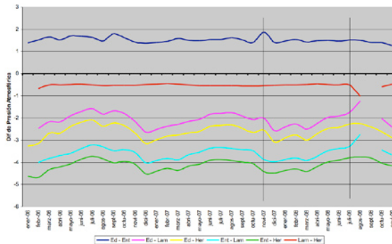
Figura 9. Comportamiento de la diferencia de presión entre las estaciones de medición, en los valores de los promedios mensuales. 9. irudia. Neurketa estazioen arteko presio aldearen jokabidea, hileroko batez bestekoen balioetan.
