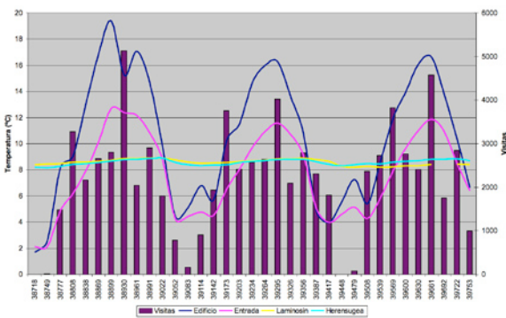
Figura 4. Comportamiento del promedio de temperaturas en las diferentes estaciones en la cueva Mendukilo, en el periodo 2006 – 2008.
