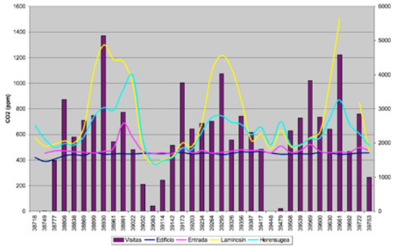
Figura 5. Comportamiento del promedio mensual del CO2 en las diferentes estaciones y su relación con el régimen de visitas.
