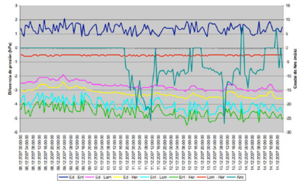
Figura 11. Comportamiento de la diferencia de presión y caudal de aire en invierno. 11. irudia. Presio aldearen eta aire emariaren jokabidea neguan.
