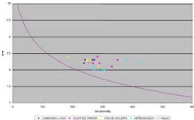
Figura 3. Relación de la conductividad eléctrica y el pH en las aguas muestreadas en la cueva Mendukilo.
